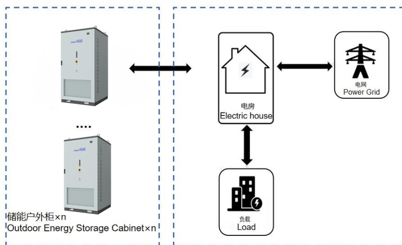
图 1-1 并网模式 Figure 1-1 Grid-side mode
